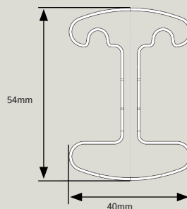
Coupe du poteau Isis®
